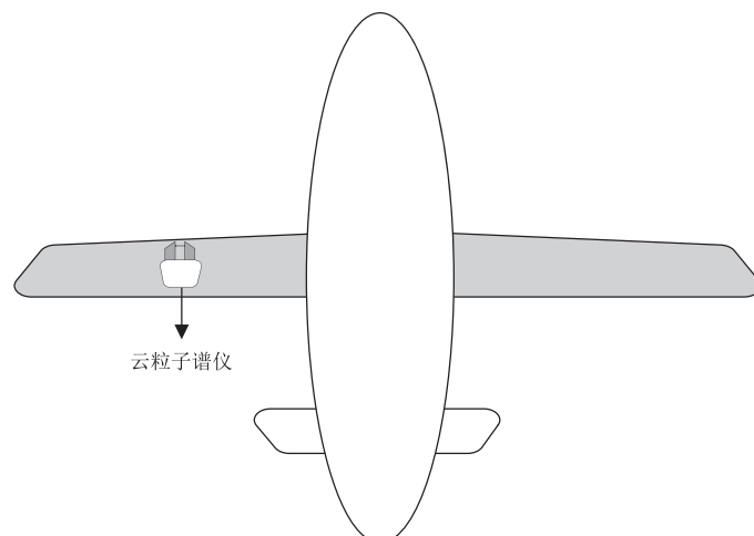
图 D.1 云粒子谱仪安装位置示意图
