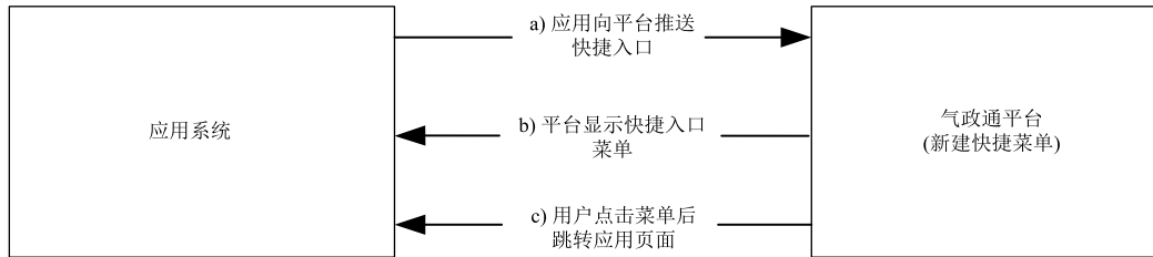
图 7 新建快捷菜单集成处理流程示意图
