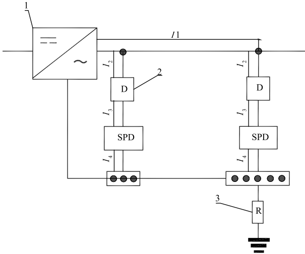
图 6 靠近逆变器交流侧的 SPD 设置图
